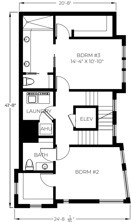
LVL 2 - 820 SF (LIVABLE)
